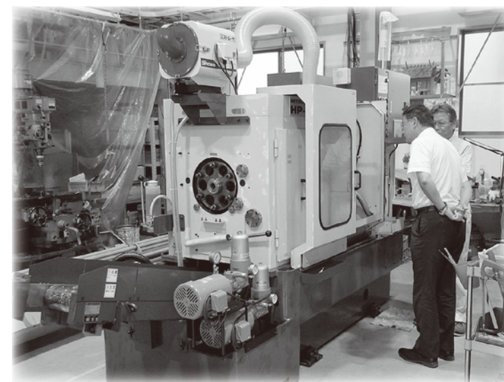
工場内で修理中の六軸自動旋盤
