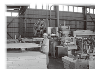
写真上:木拾い作業 写真下:プレカット加工は使用目的別の機器で全てコンピューター制御により全自動で稼働しています。
